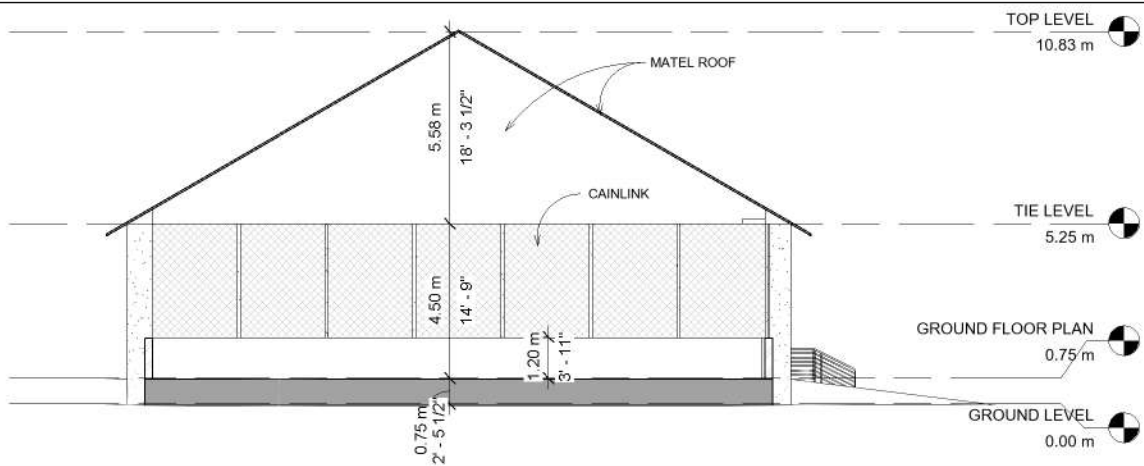
1 Section 1 1 : 110
